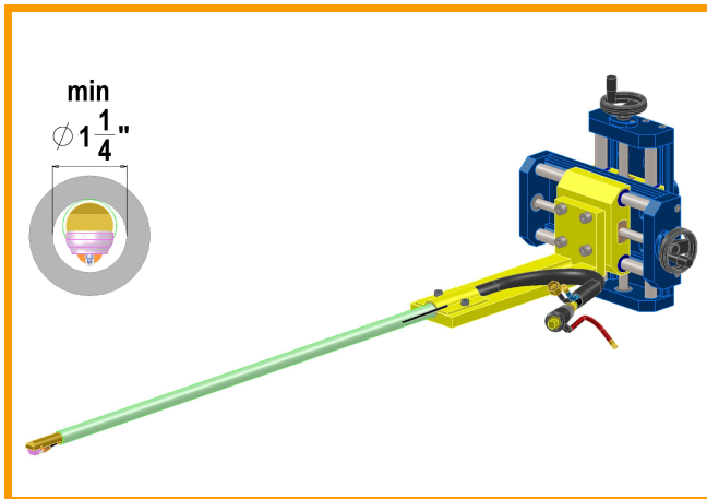
TIG 32 LONGITUDINALE
