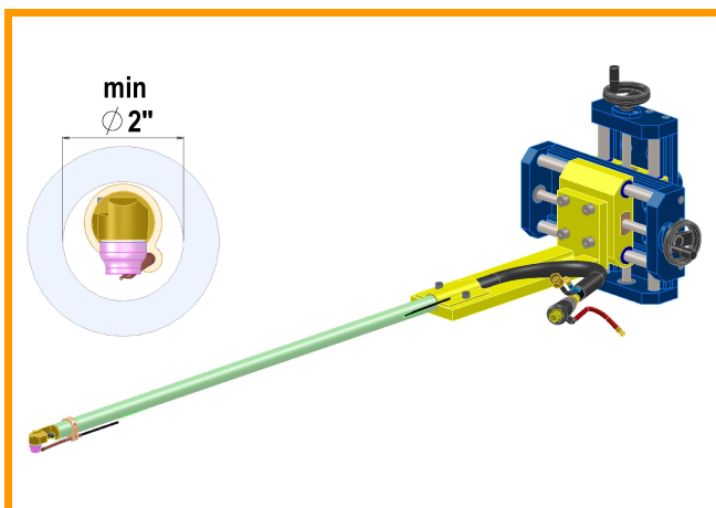
TIG 51 CIRCONFERENZIALE
