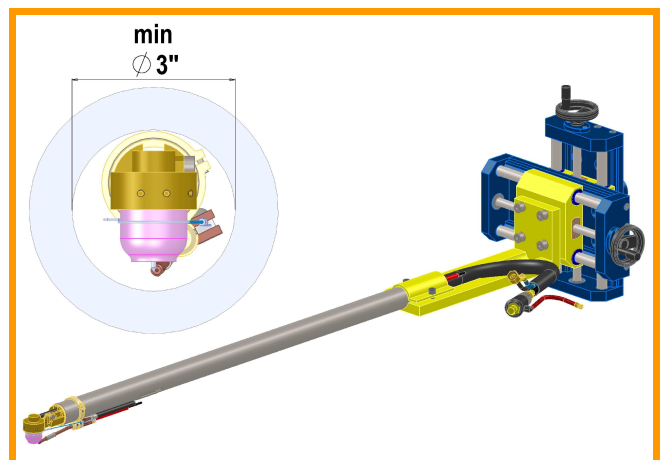
TIG 76 CIRCONFERENZIALE FILO CALDO o FREDDO
