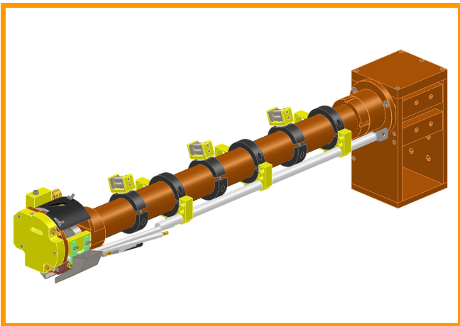
TORCIA NASTRO 30 PER INTERNI CIRCONFERENZIALE
