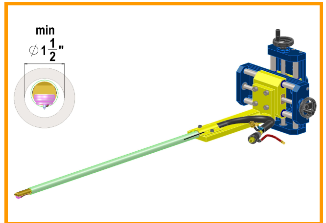
TIG 38 CIRCONFERENZIALE o LONGITUDINALE
