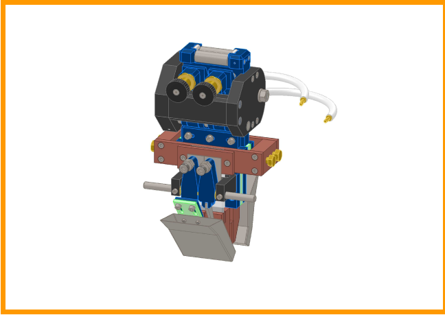
TORCIA NASTRO 60-30
